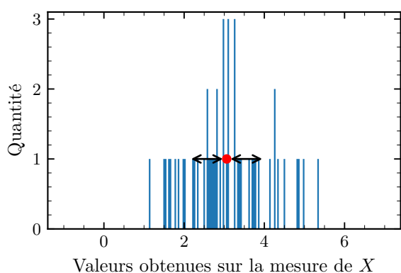
(a) Dispersion des mesures d'une grandeur X de moyenne \bar{X} = 3,06 (point rouge) et d'écart-type \sigma_s = 0,982 (largeur d'une double flèche).
