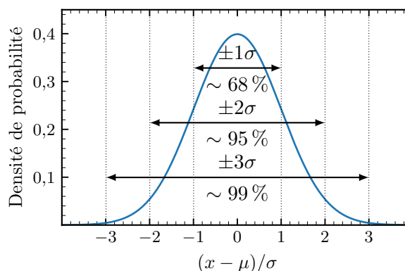
(b) Cas d'une distribution suivant la loi normale.
