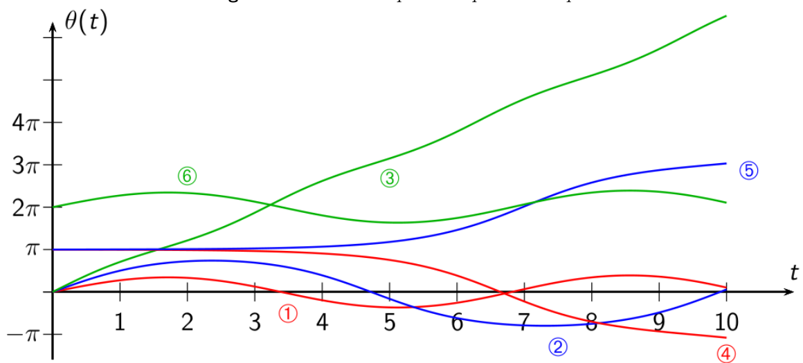
Figure 4 – Évolution de \theta pour le pendule simple.
