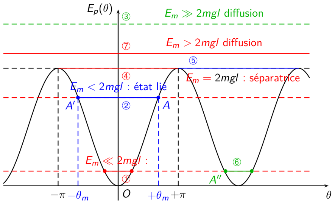
Figure 2 – Energie potentielle dans le cas du pendule simple.
