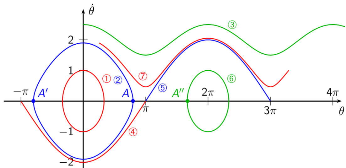
Figure 3 – Portrait de phase du pendule simple.
