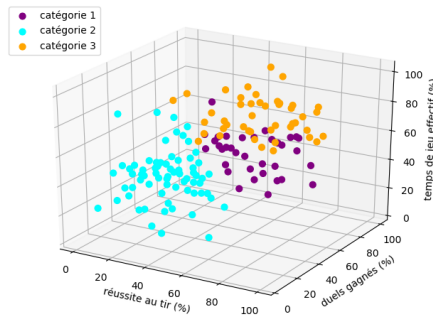
résultat de l'algorithme des k -moyennes avec k = 3 , étudiant(e)1
