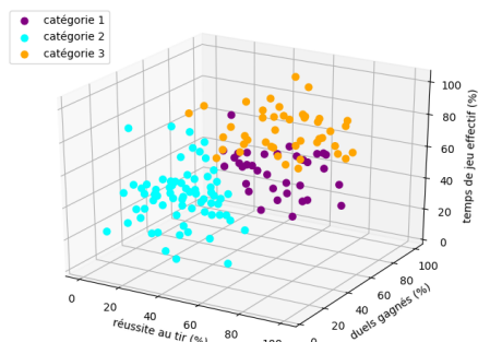
résultat de l'algorithme des k -moyennes avec k = 3 , étudiant(e)1
