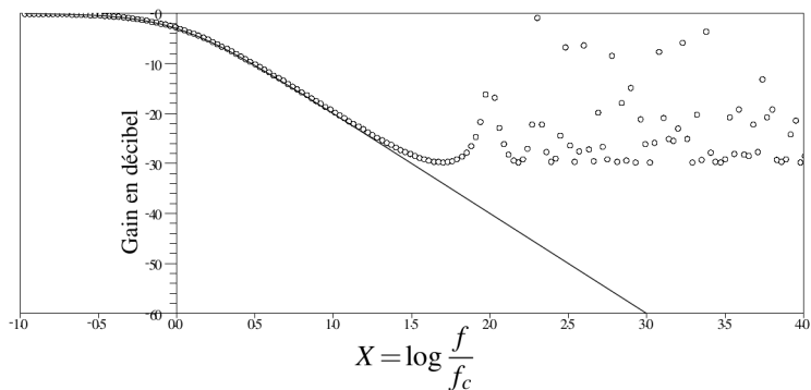
Figure 5.13 – Courbe de réponse en gain du filtre numérique passe-bas d'ordre 1 avec f_e = 10 kHz.
