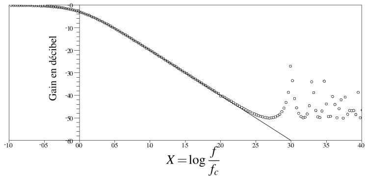
Figure 5.14 – Courbe de réponse en gain du filtre numérique passe-bas d'ordre 1 avec f_e = 100 kHz.
