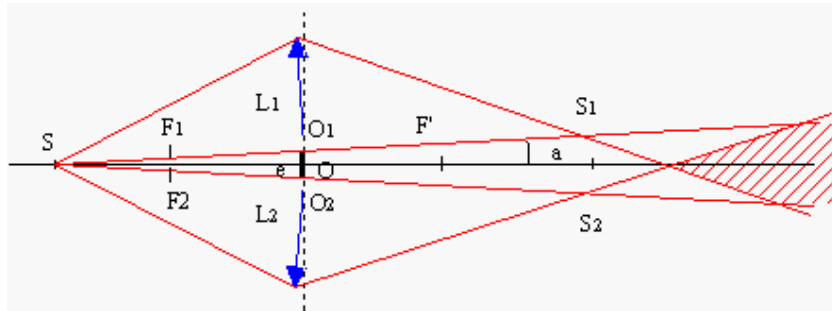
FIGURE 1 – Bientille de Billet
