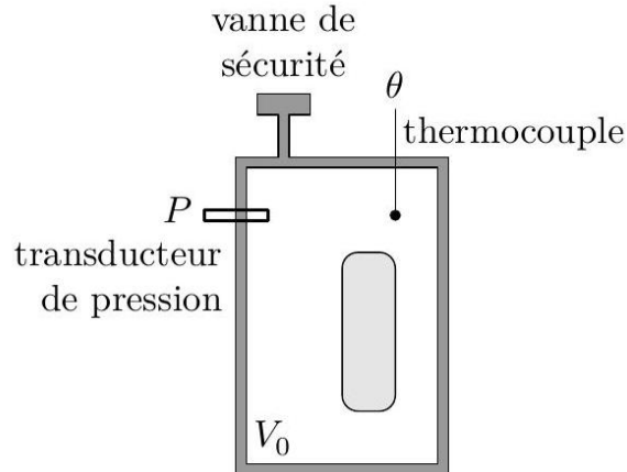
Figure 3 Vent Sizing Package 2 (VSP2™), calorimètre adiabatique à faible inertie thermique, d'après https://www.fauske.com
