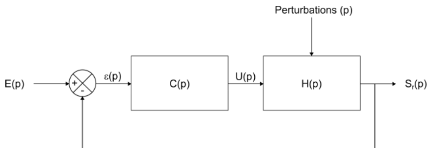
Figure 2 : Schéma bloc modélisant le système. E(p) représente l'entrée, S(p) la sortie, U(p) la commande, Perturbations (p) les perturbations appliquées au système, \varepsilon(p) l'erreur, H(p) le système et C(p) le correcteur. p représente la variable de Laplace.
