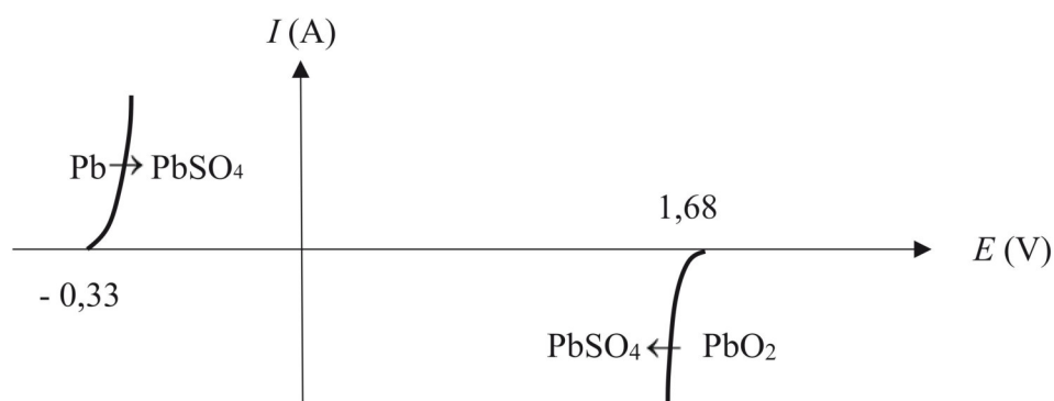
Figure 5 – Courbes intensité-potentiel
